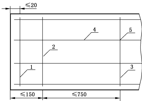
a) 网片构造示意图
